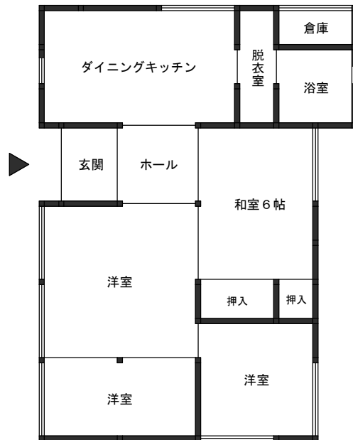
1階平面図 (離れ)
