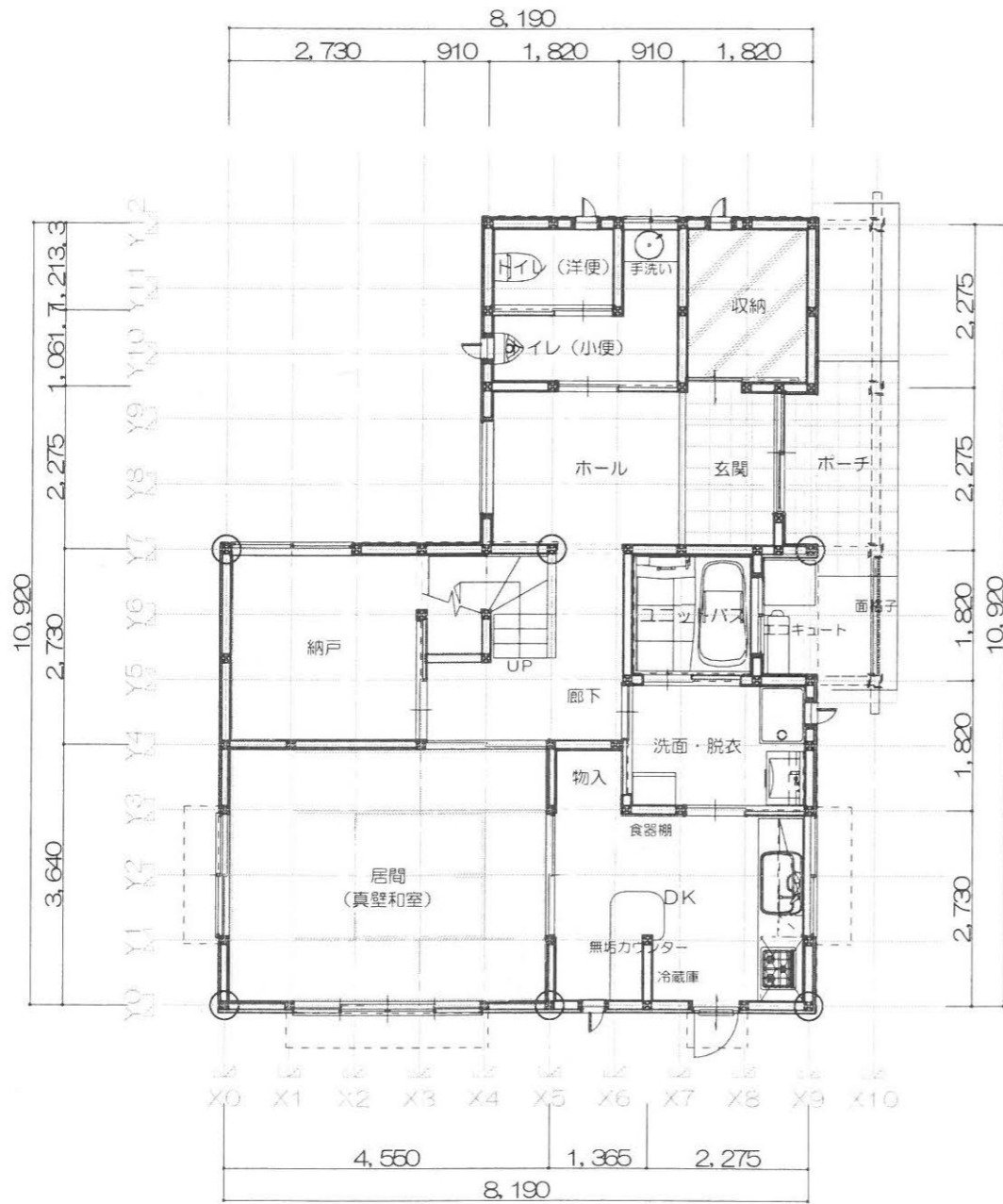
平面詳細図 1階
