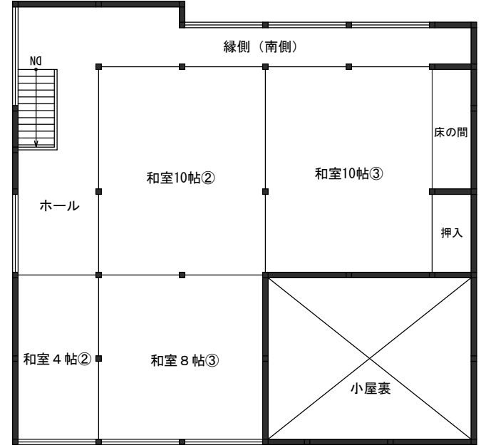
2 階平面図
