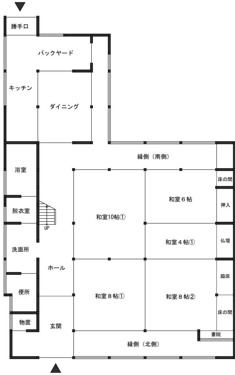
1 階平面図
